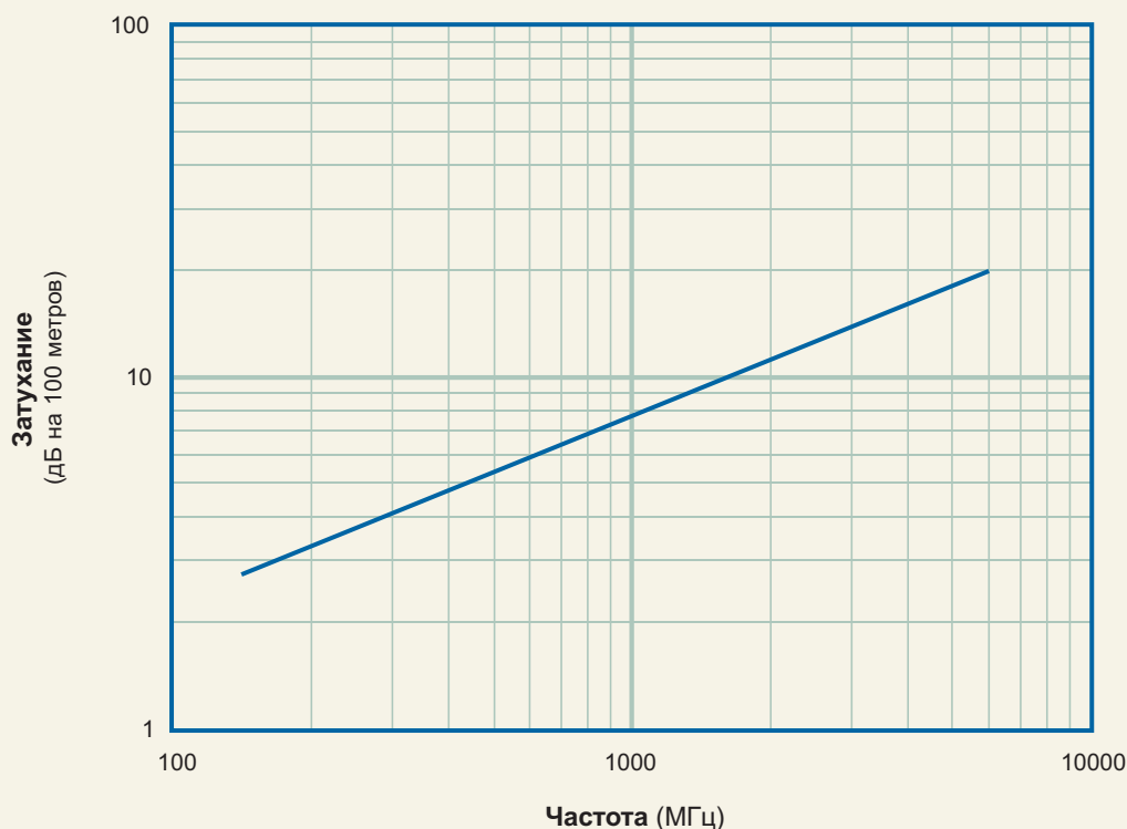
Типовое затухание PK 50-12-33 (1/2" Feeder Cable)
